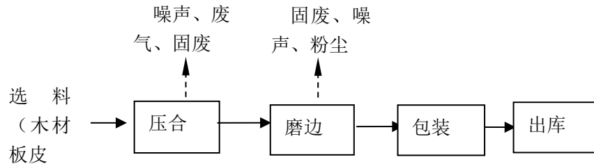
图1 项目生产工艺及产污流程图
