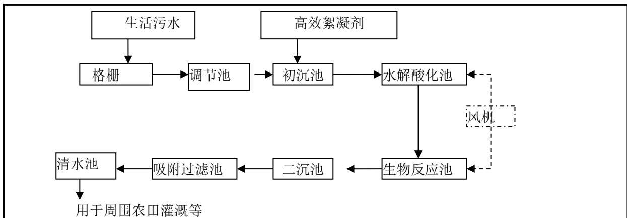
图 6 污水处理厂工艺流程图
