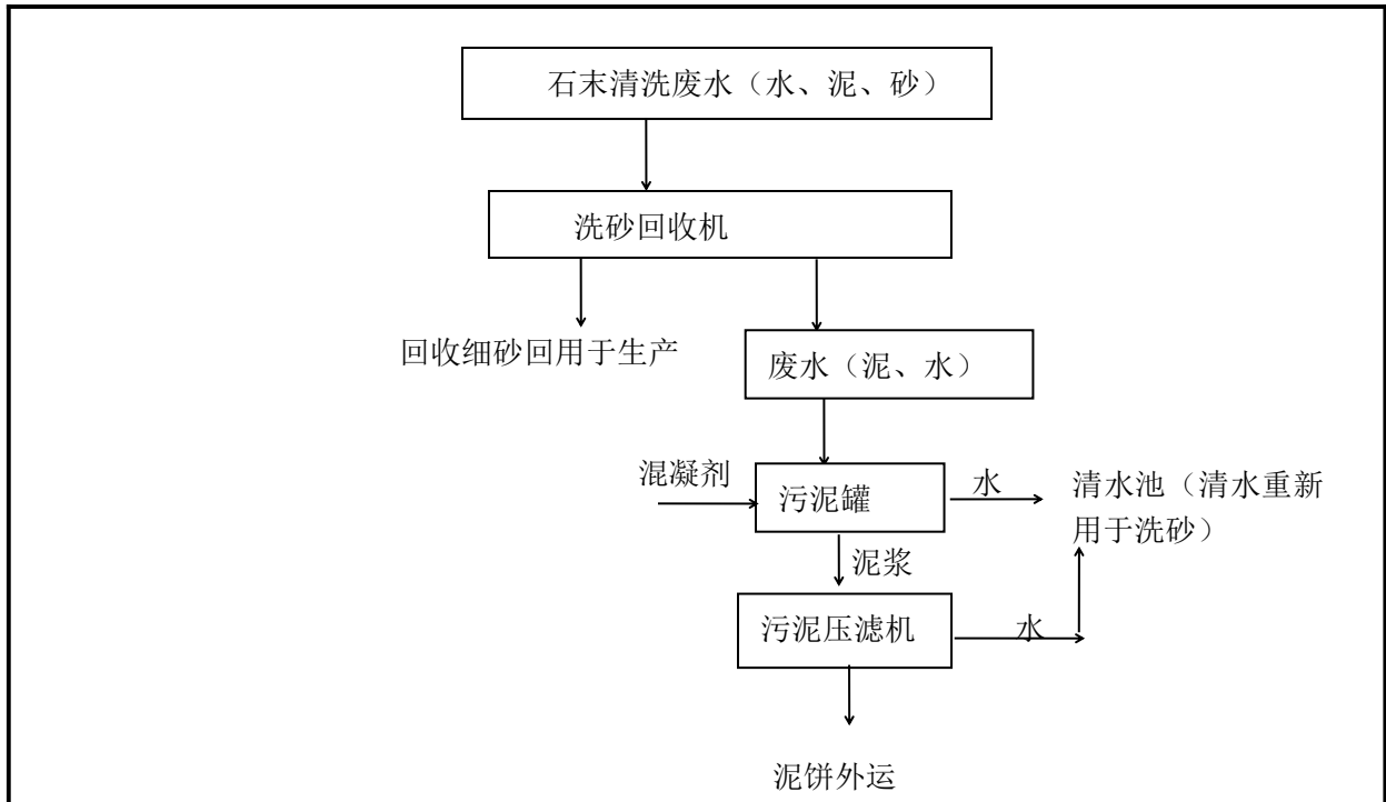
图 5 项目石末清洗废水处理流程图
