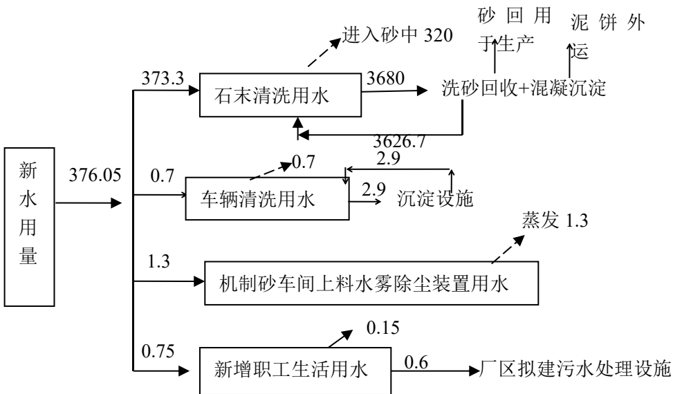
图 1 扩建项目水平衡图 单位： t/d
