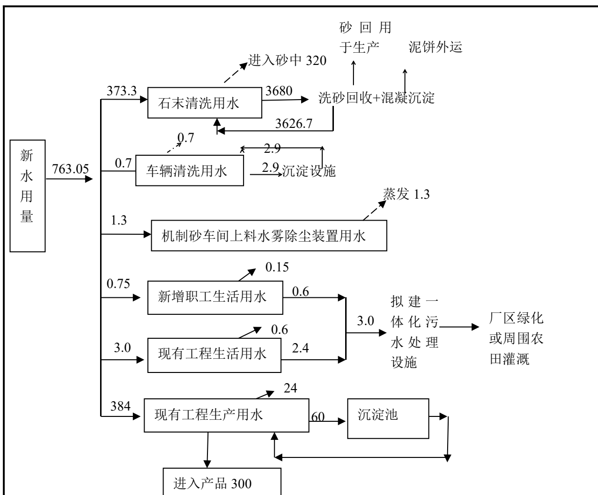
图 2 扩建项目完成后厂区整体工程项目水平衡图 单位: t/d
