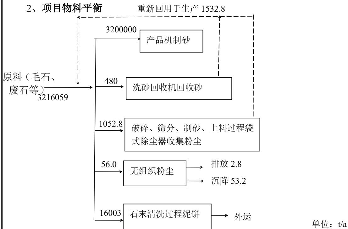
图 4 项目物料平衡图
