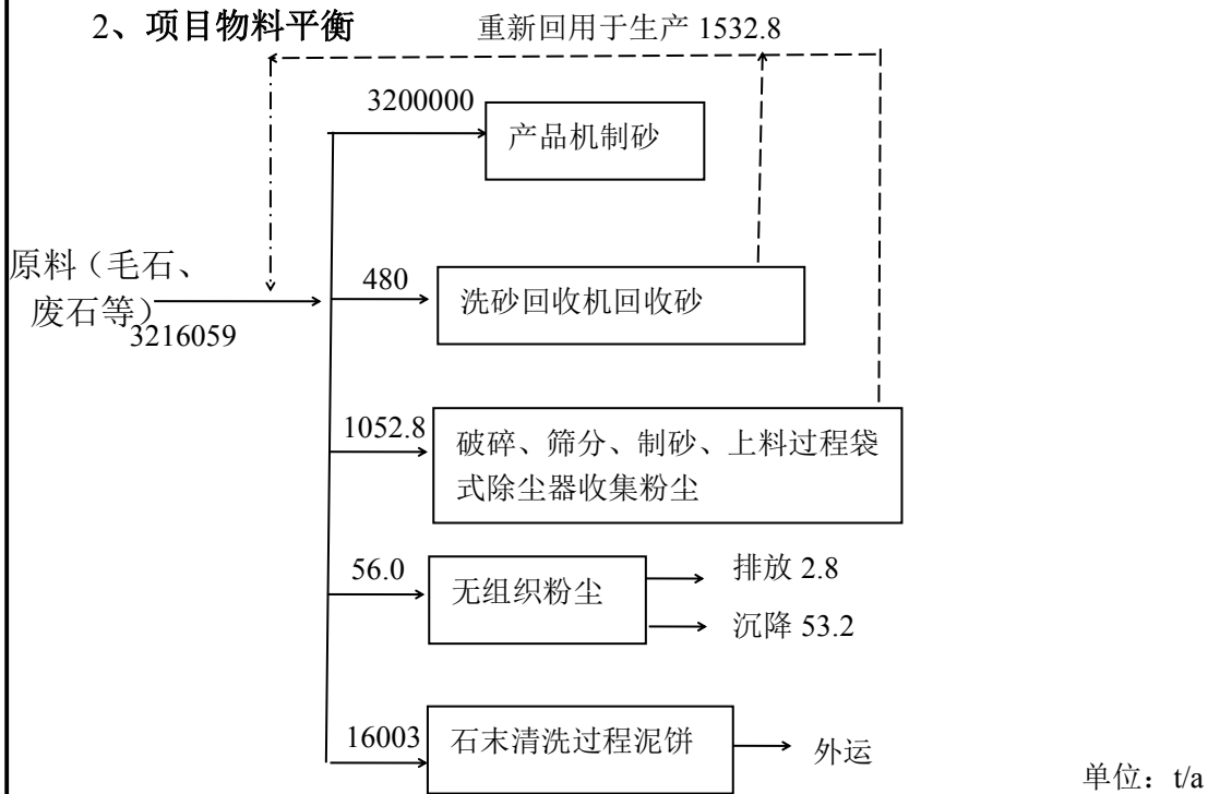
图 3 项目物料平衡图
