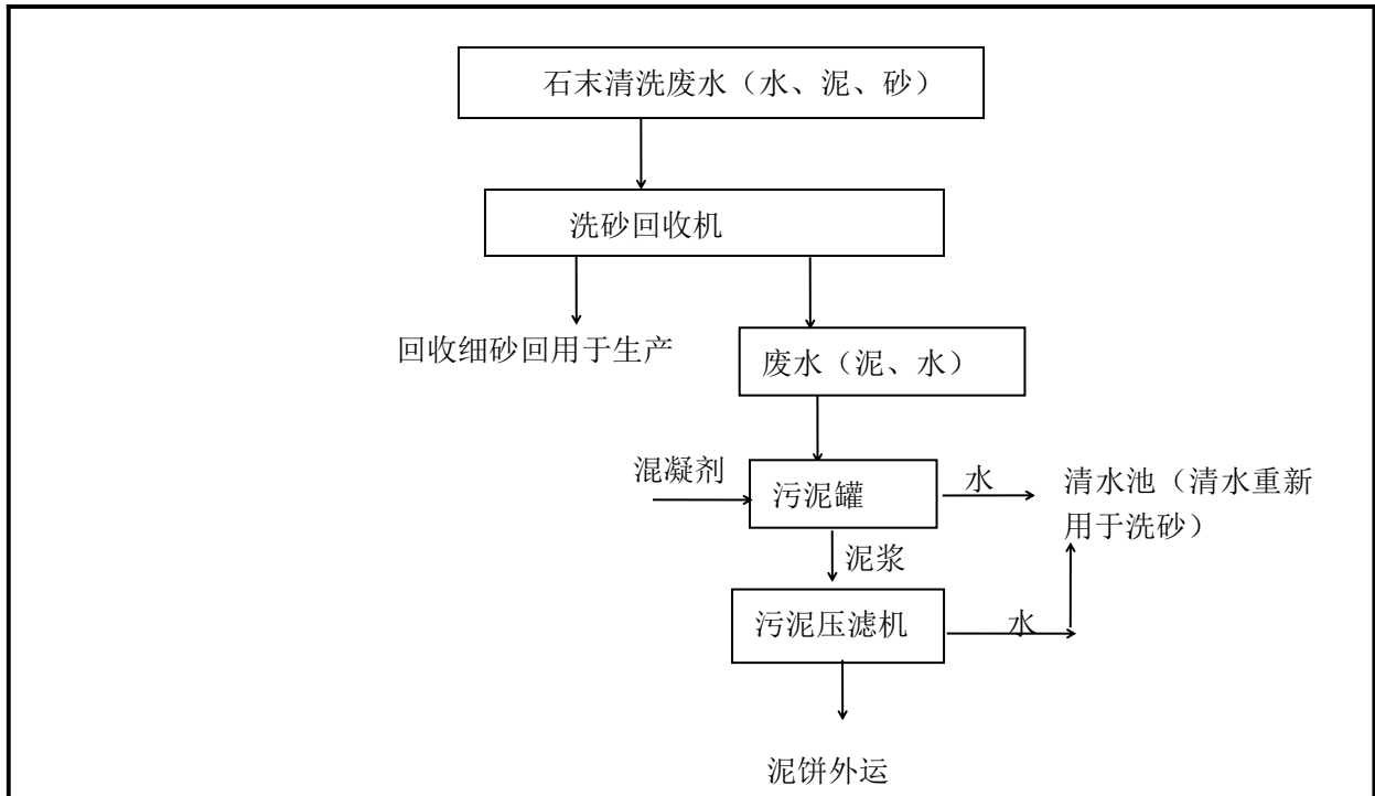
图 4 项目石末清洗废水处理流程图
