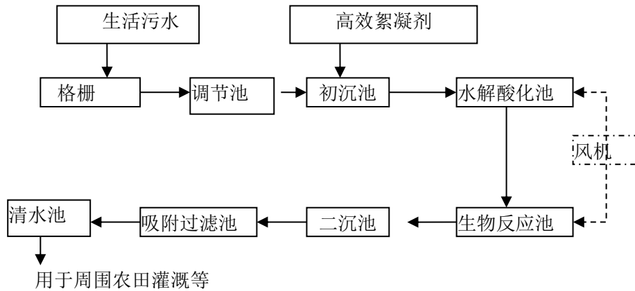
图 5 项目生活污水处理工艺流程图
